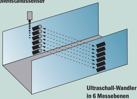
Höhenstandssensor
